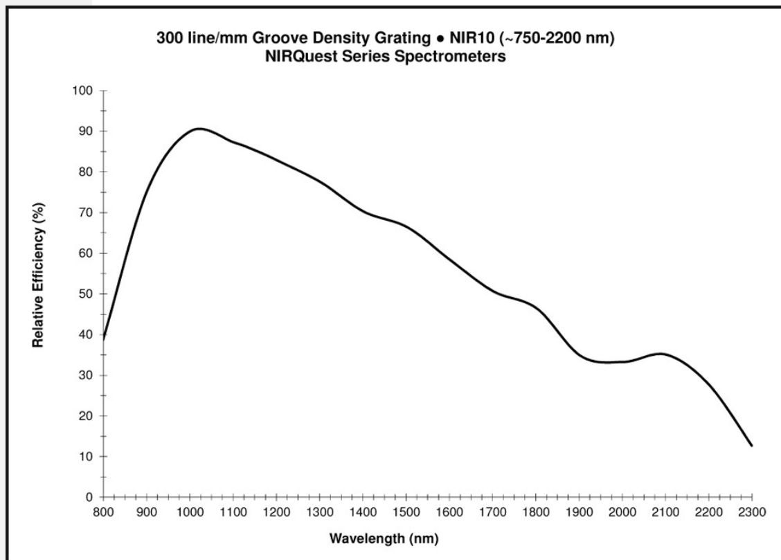
グレーティング NIR10 (300 Lines/mm)
