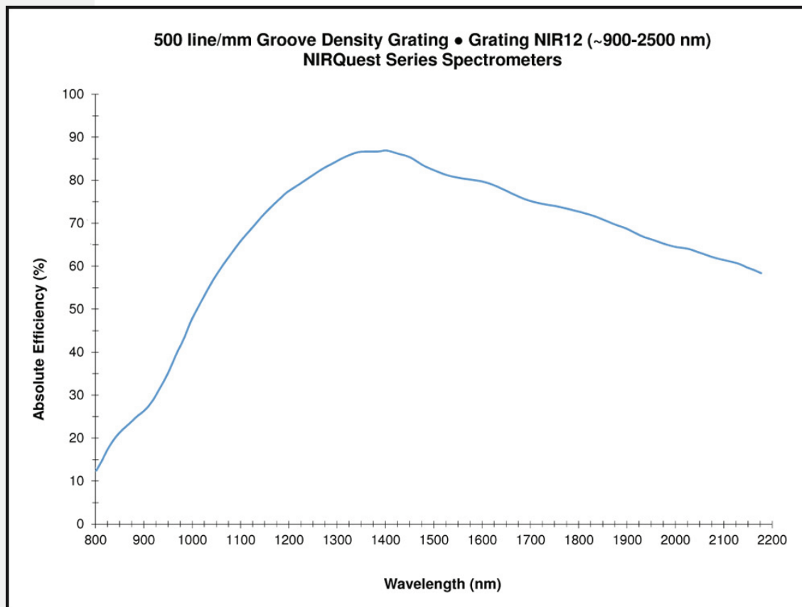
グレーティング NIR12 (500 Lines/mm)
