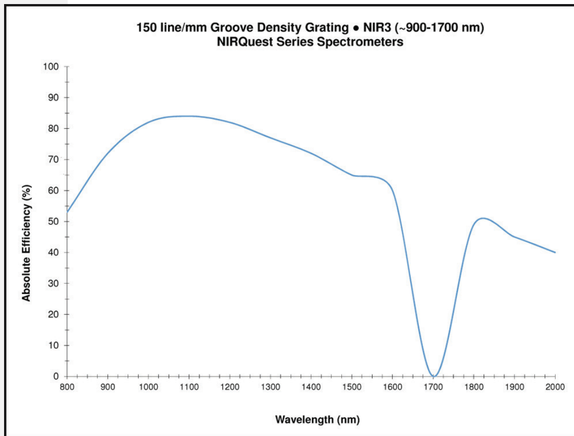
グレーティング NIR3 (150 Lines/mm)
