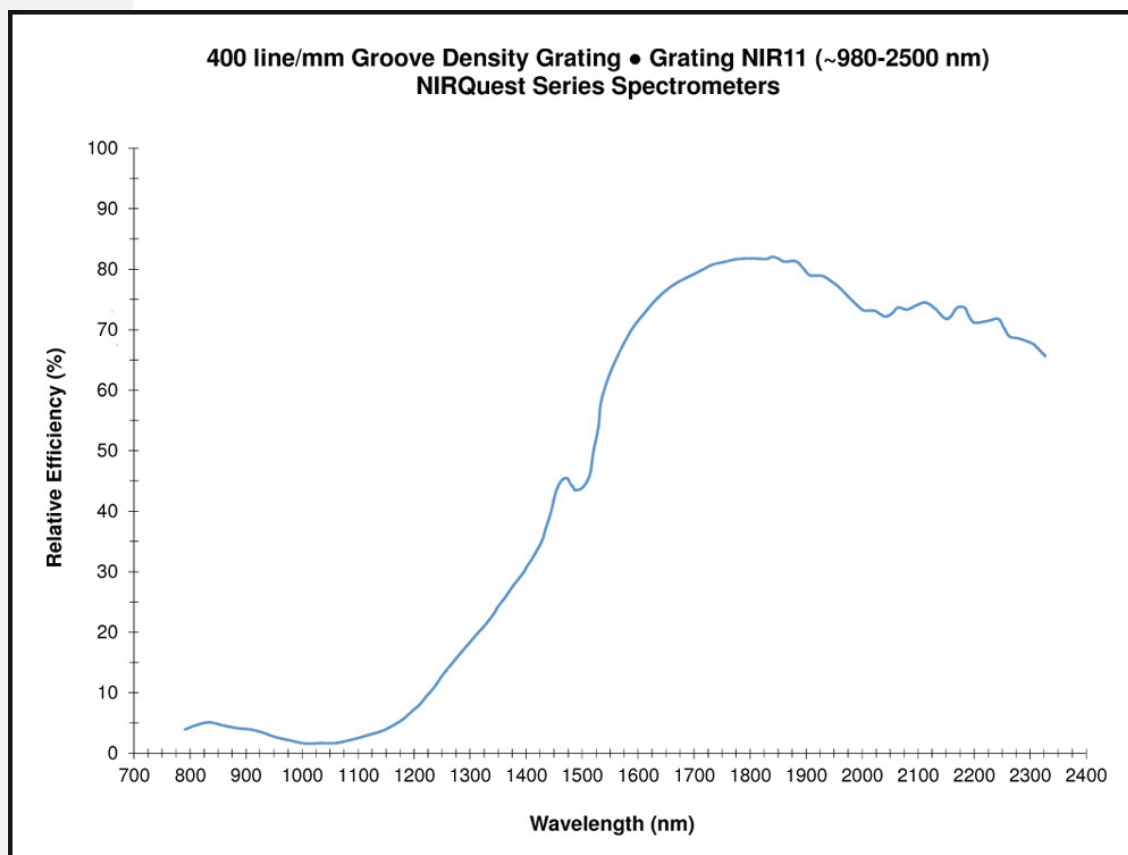
グレーティング NIR11 (400 Lines/mm)
