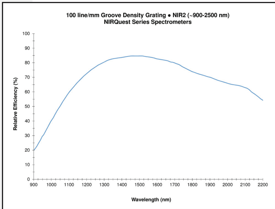
グレーティング NIR2 (100 Lines/mm)
