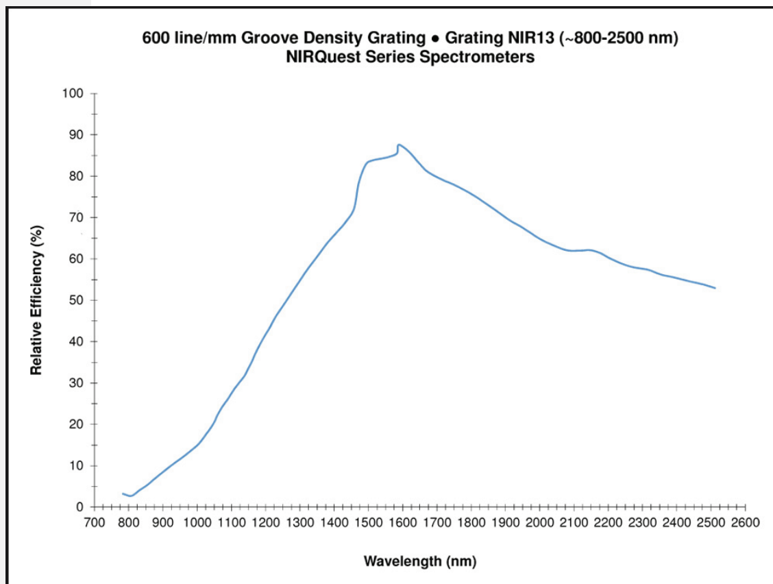
グレーティング NIR13 (600 Lines/mm)
