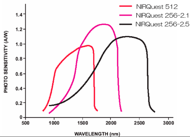
NIRQuest シリーズ (HAMAMATSU G9204-512 / G9206-256 / G9208-256)
