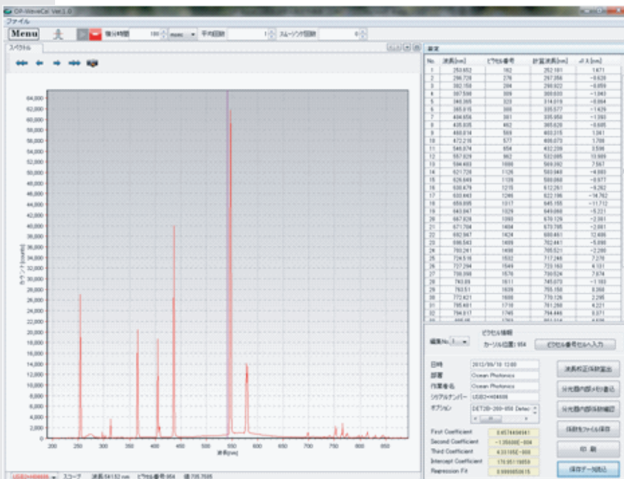
HG-2 波長校正水銀アルゴン光源
